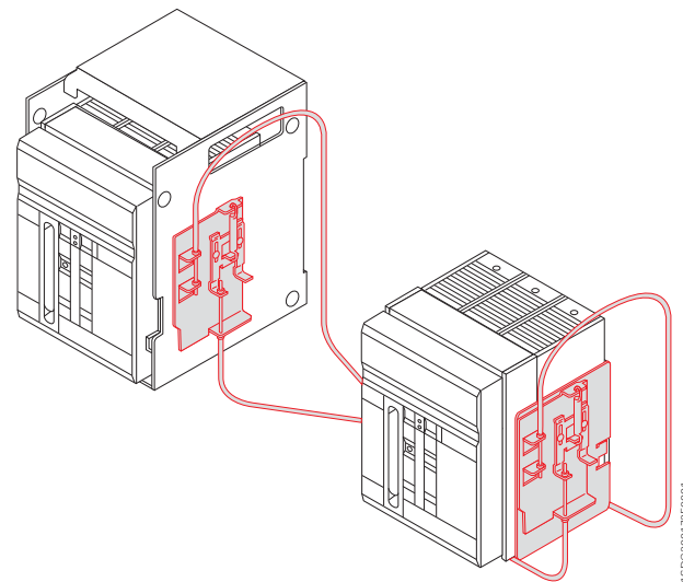
Horizontal interlock
