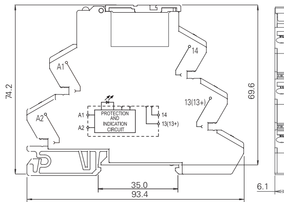
RV8S-S Spring Clamp Terminal (mm)
