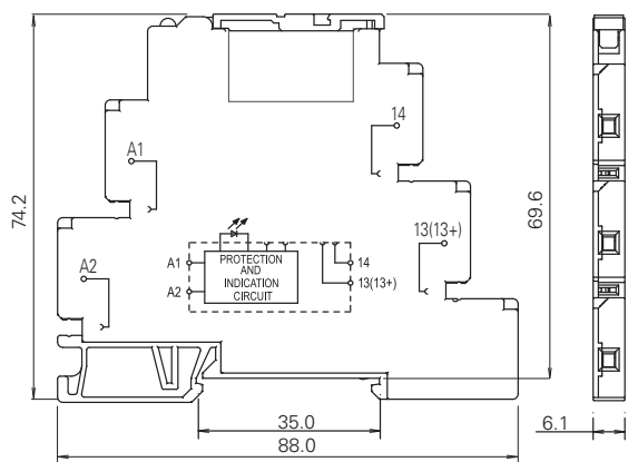
RV8S-L Screw Terminal (mm)
